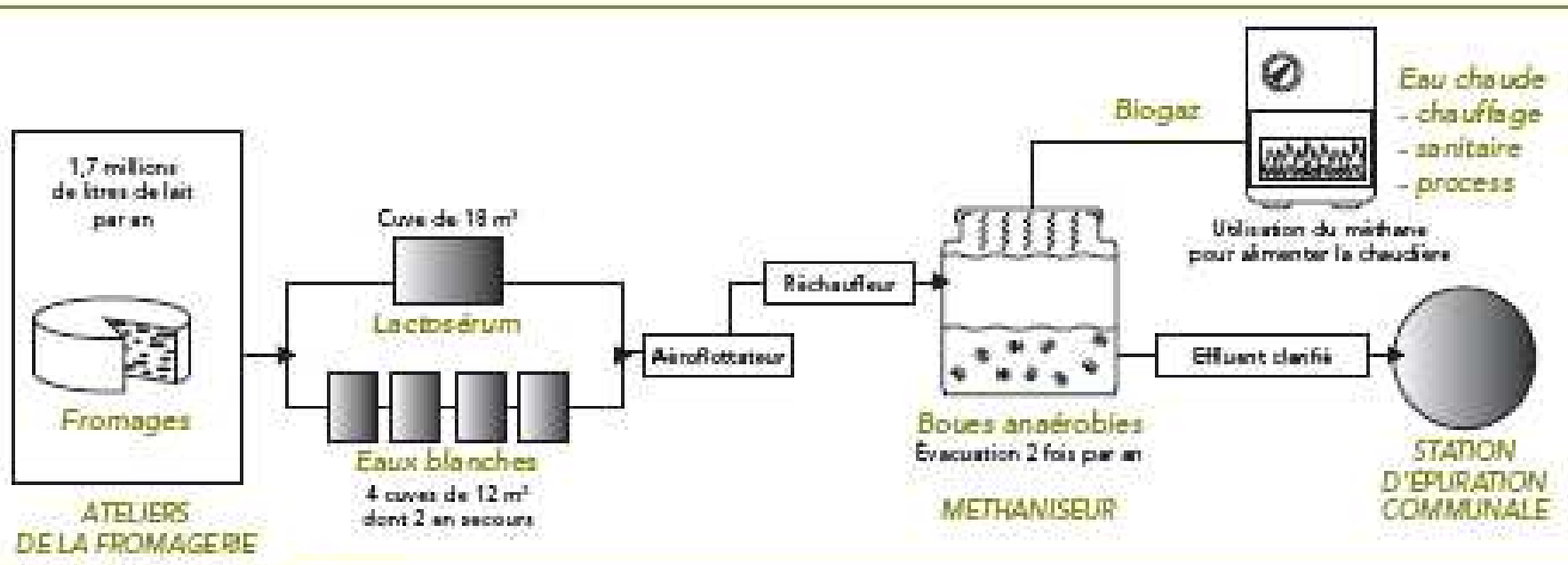
Schéma : Traitement par méthanisation.
